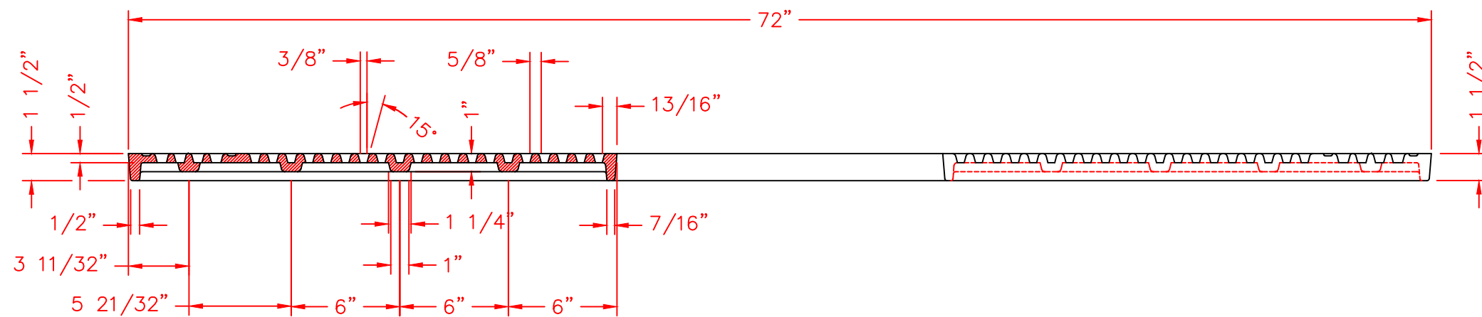
SECTION A-A
