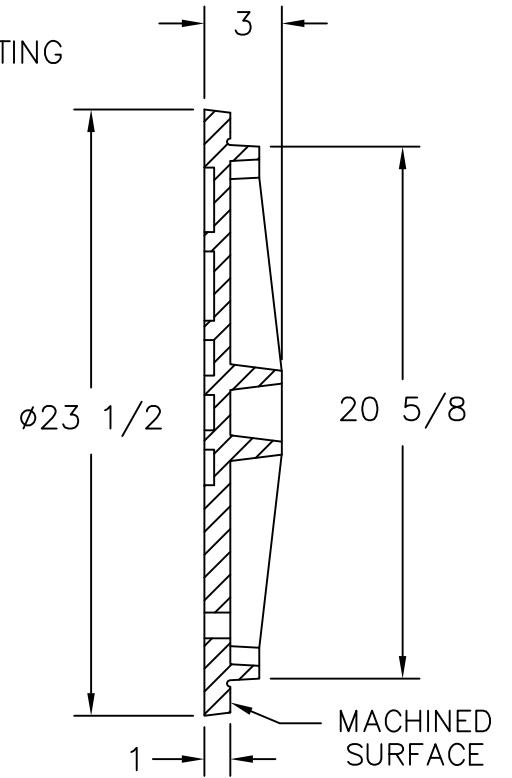
SECTION A-A (Cover)
