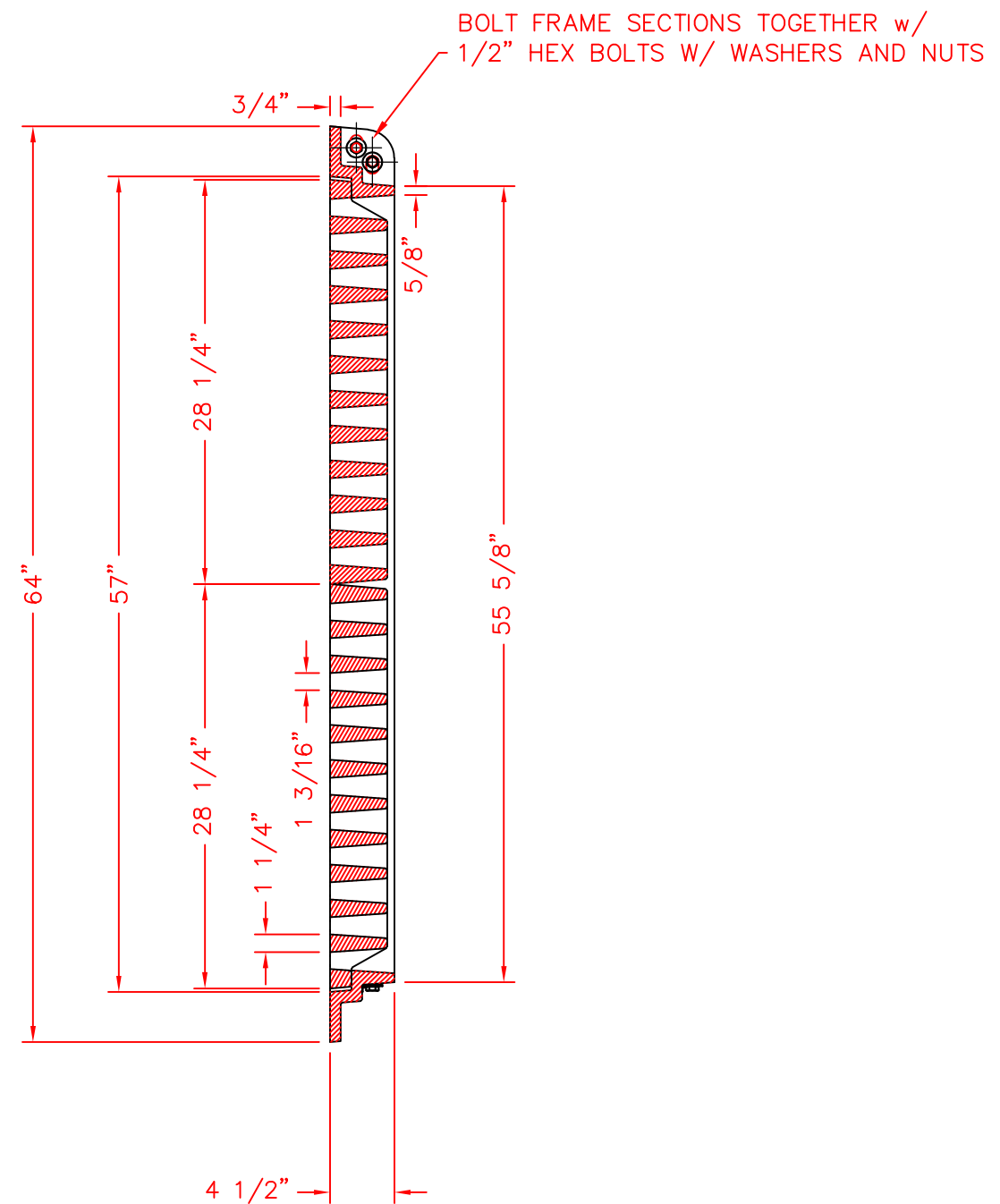
SECTION A-A
