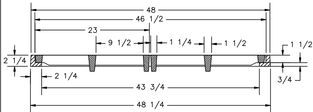
A-A SECTION
