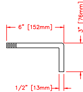
ANCHOR BOLT DETAIL (SCALE: 1=4)
