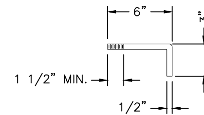
ANCHOR STUD DETAIL
