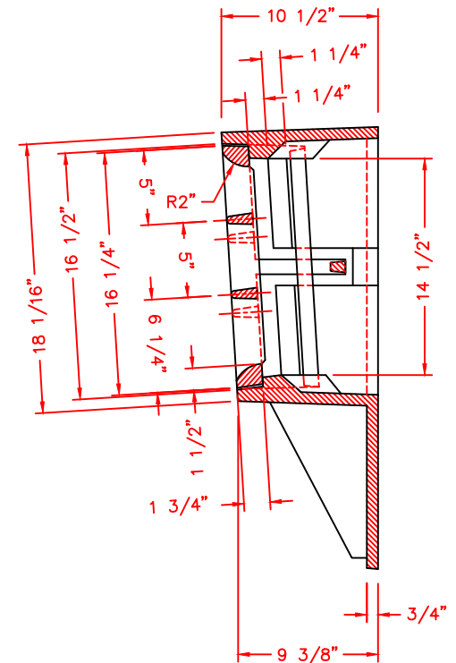
SECTION A-A
