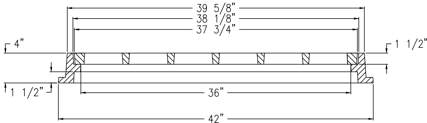
SECTION A-A
